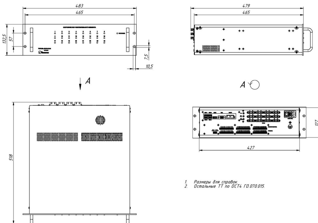
Рисунок 1 - Габаритный чертеж БОС
